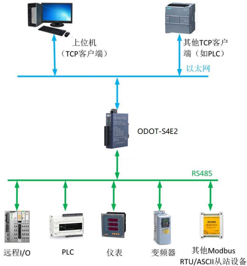
图 3.1 系统拓扑图
